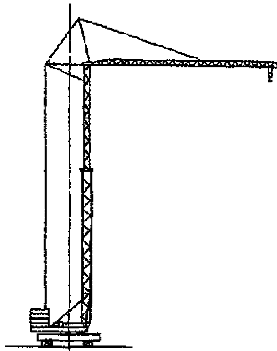
Gru a rotazione in basso
